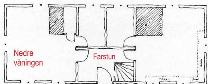
Ritning 4 maj 1986 från skiss nedtecknad 28 april 1986 i samband med fotografering av bilderna ovan. Måtten är ej exakt uppmätta. Skissen visar översiktligt rumsindelning samt placering av spisar, plåtugnar, dörrar och fönster. I nedre våningens stora rum till höger fanns väggfasta bänkar längs två väggar. / Göran Strömfors
